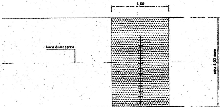
scavo trasversale alla carreggiata
